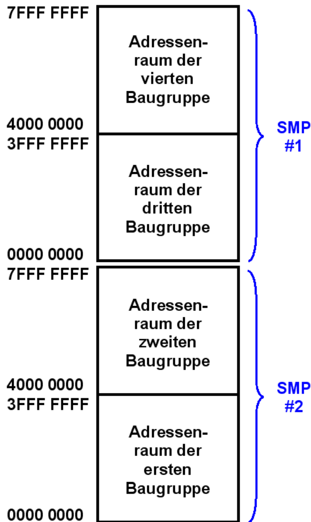
Abb. 12.1.3 NUMA Adressenraum
