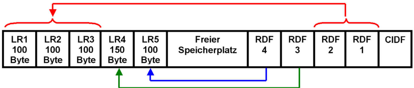
Abb. 6.2.7 Aufeinanderfolgende (contiguous) Records mit identischer Länge
