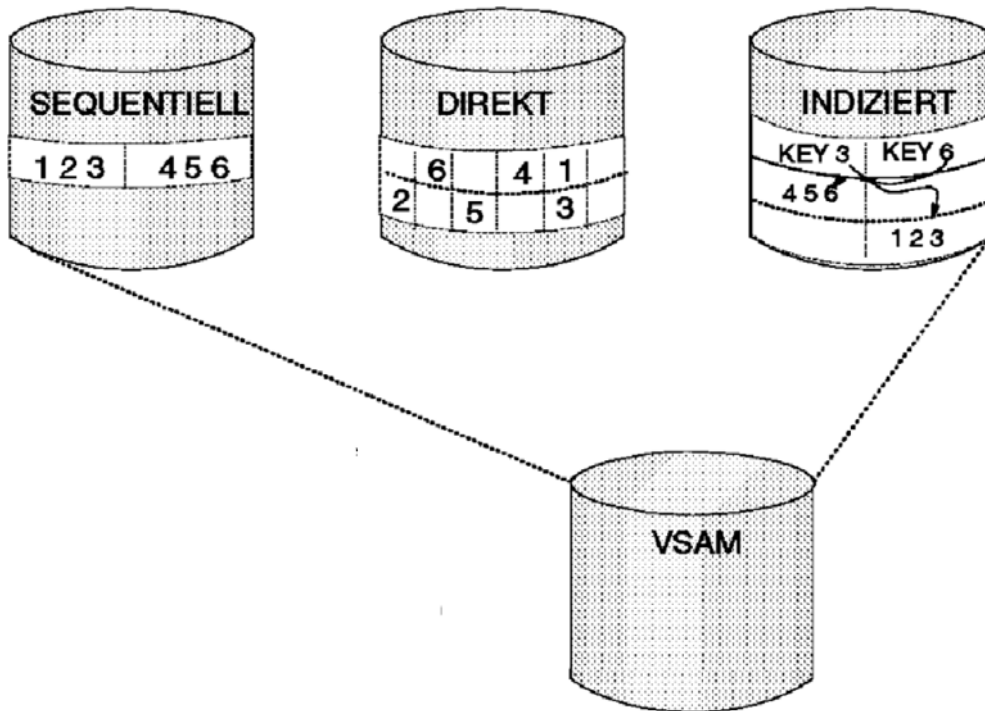
Abb. 6.2.2 Unterschiedliche Arten von VSAM Datasets
